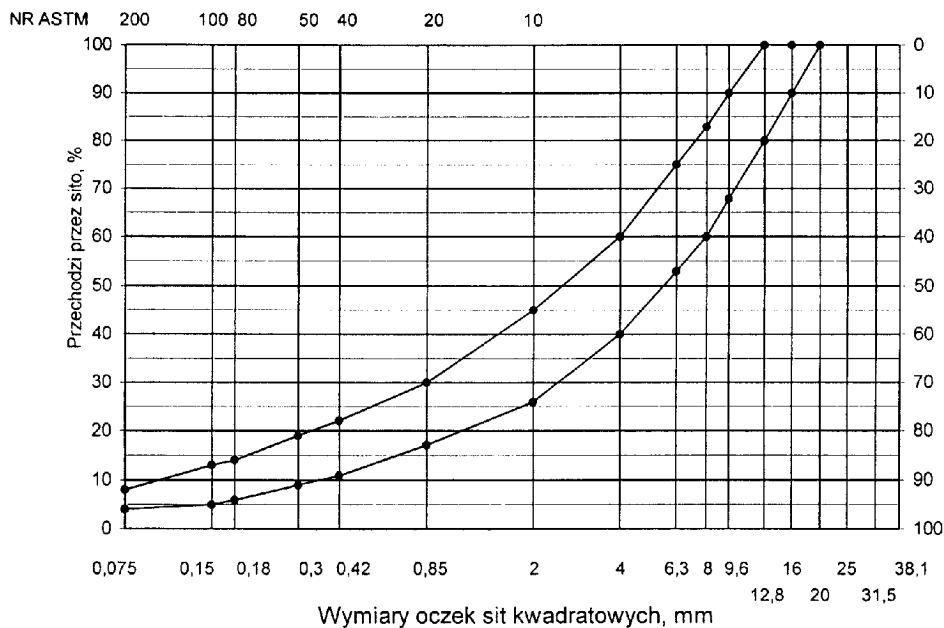
Rys. 4. Krzywe graniczne uziarnieni a mieszanki mineralnej BA od 0 do 16 mm do podbudow y nawierzchni drogi o obciążeni u ruchem KR 1 lub KR 2
