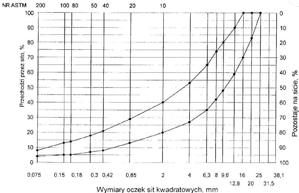
Rys. 3. Krzywe graniczne uziarnienia mieszanki mineralnej BA od 0 do 20 mm do podbudowy nawierzchni drogi o
