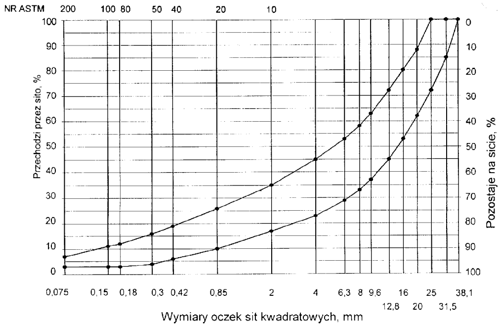
Rys.1. Krzywe graniczne uziarnienia mieszanki mineralnej BA od 0 do 31,5 mm do podbudowy nawierzchni drogi o obciążeniu
