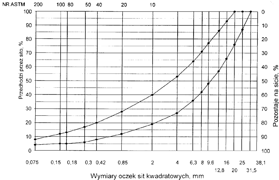
Rys. 2. Krzywe graniczne uziarnienia mieszanki mineralnej BA od 0 do 25mm do podbudowy nawierzchni drogi o obciążeniu u ruchem KR 1 lub KR 2
